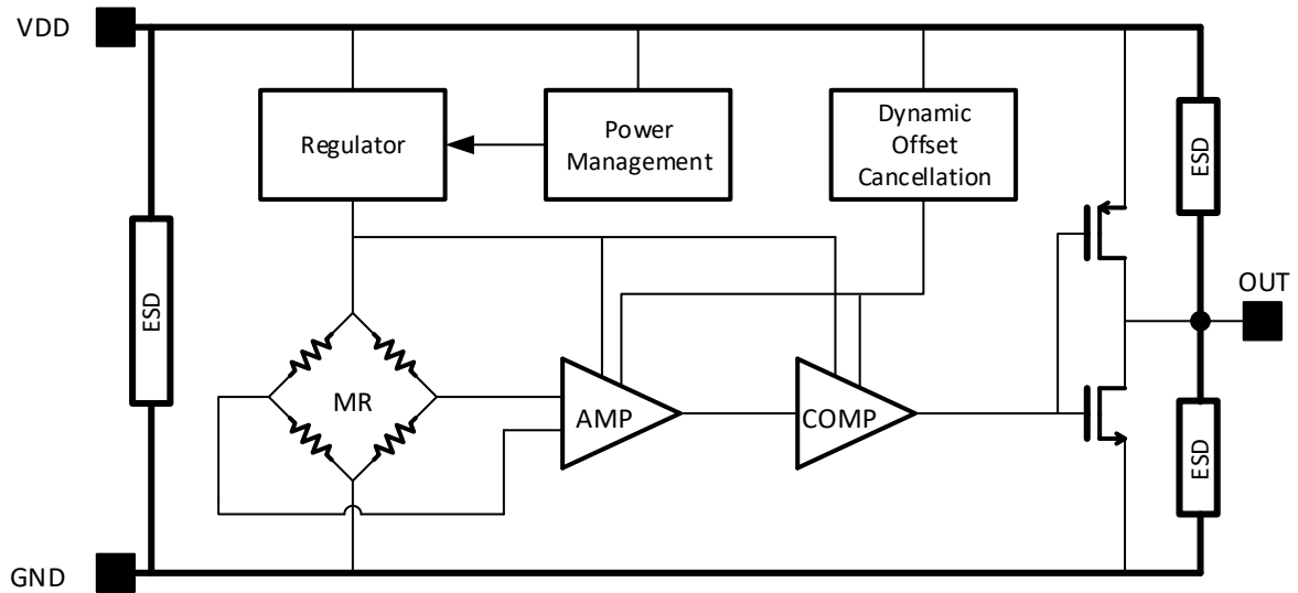
图 1 模块/线路图
